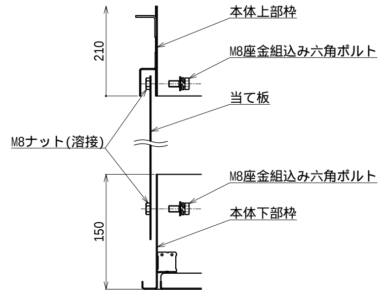
ジョイント部詳細図
